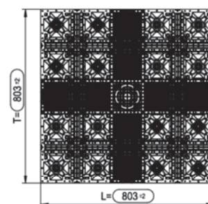
Figure 1e– Caractéristiques dimensionnelles du module Rigofill ST
