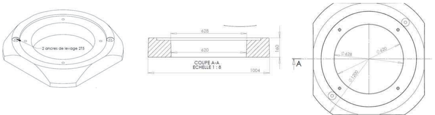
Figure 6 – Vue en coupe joint rehausse – dalle de répartition
