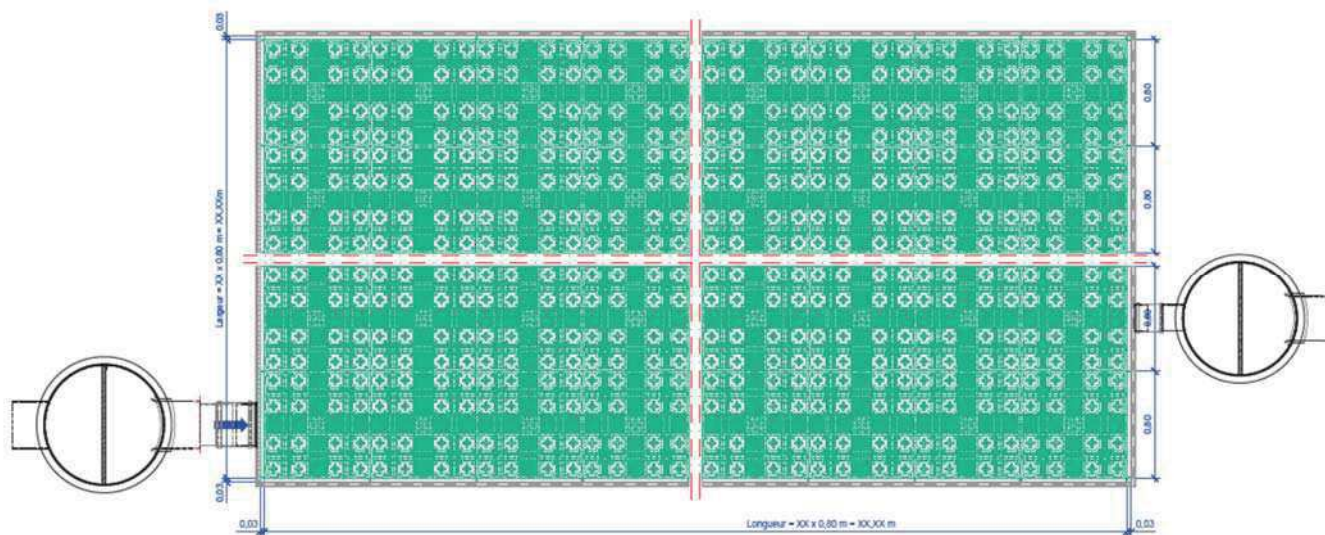
9a – Vue du haut d'un bassin réalisé avec Rigofill ST (regards externes)
