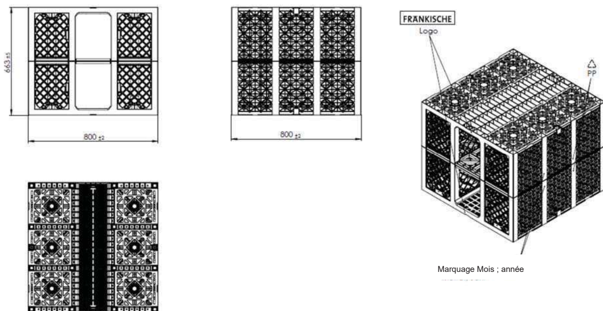
Figure 1 b- Caractéristiques dimensionnelles du module Rigofill inspect
