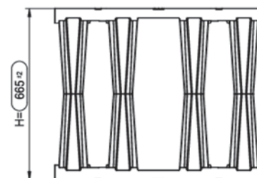
Figure 1e– Caractéristiques dimensionnelles du module Rigofill ST
