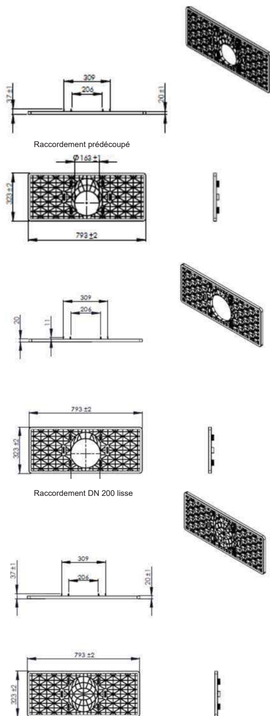
Figure 3a : Plaque d'about et plaque d'about ajourée ouverture DN 150 ou DN 200 pour Rigofill inspect
