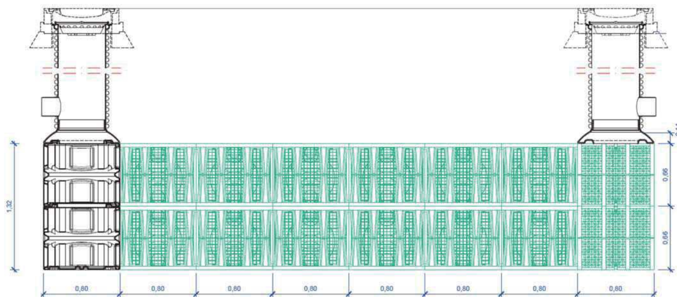
Figure 11b – Coupe de principe d'un bassin réalisé en mix Rigofill inspect et ST avec boîte d'inspection intégrée
