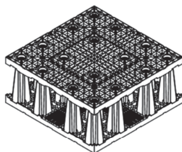
Figure 1e– Caractéristiques dimensionnelles du module Rigofill ST
