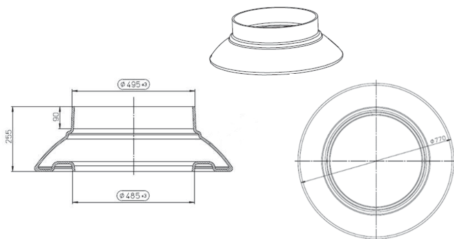
Figure 4c – Boîte d'inspection Quadro-control : cône pour rehausse
