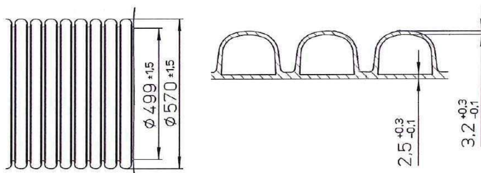
Figure 5 – Vue en coupe de la rehausse
