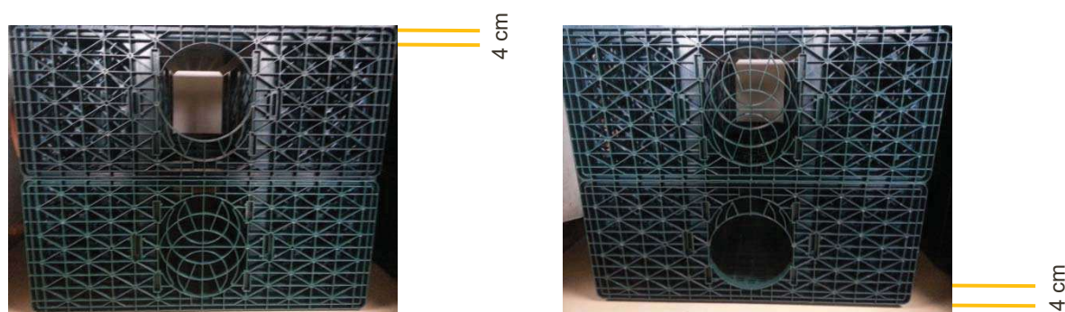
Figure 1 : Positionnement de la plaque d'about pour le passage de l'introduction (à gauche), pour le passage de la sortie (à droite)
