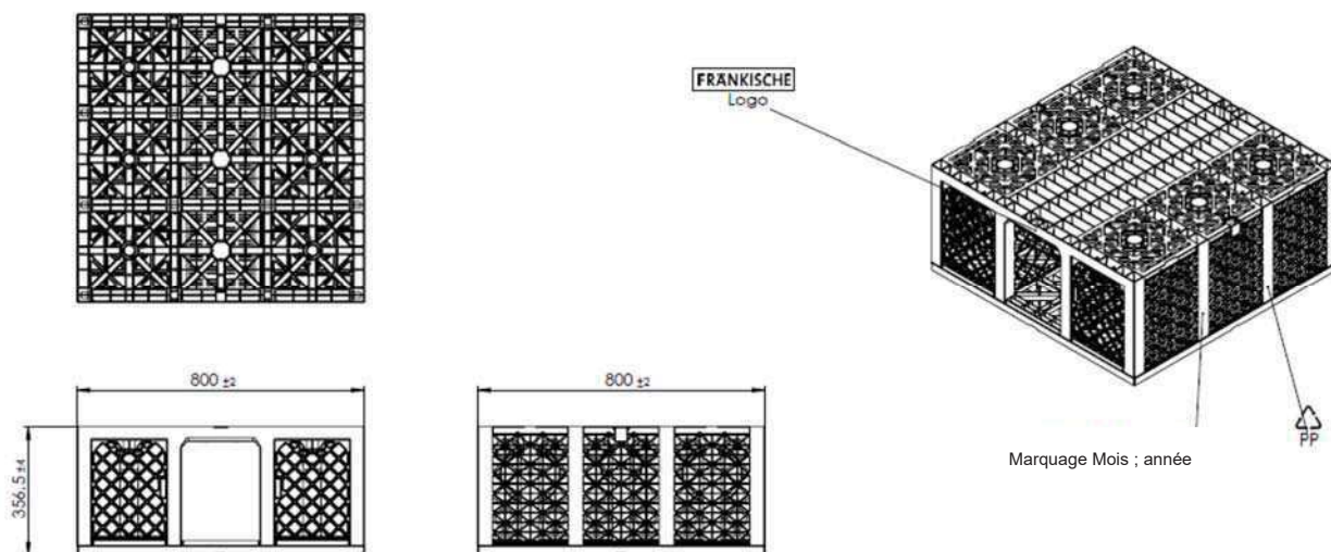
Figure 1 C- Caractéristiques dimensionnelles du demi-module Rigofill inspect
