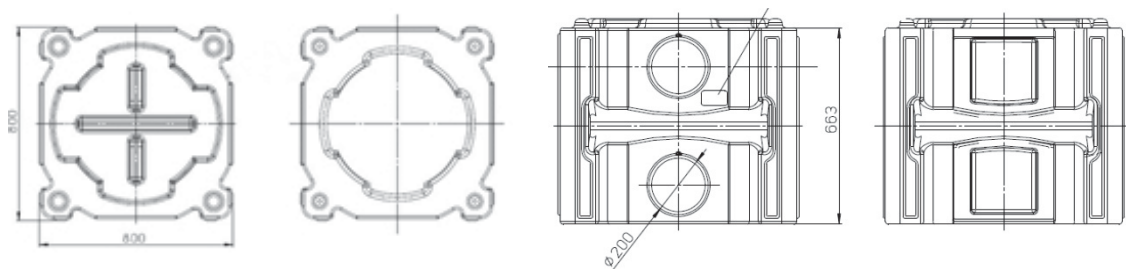
Figure 4a – Boîte d'inspection Quadro-control pour module entier
