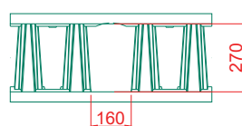
Figure 1f– Caractéristiques dimensionnelles du demi-module Rigofill ST
