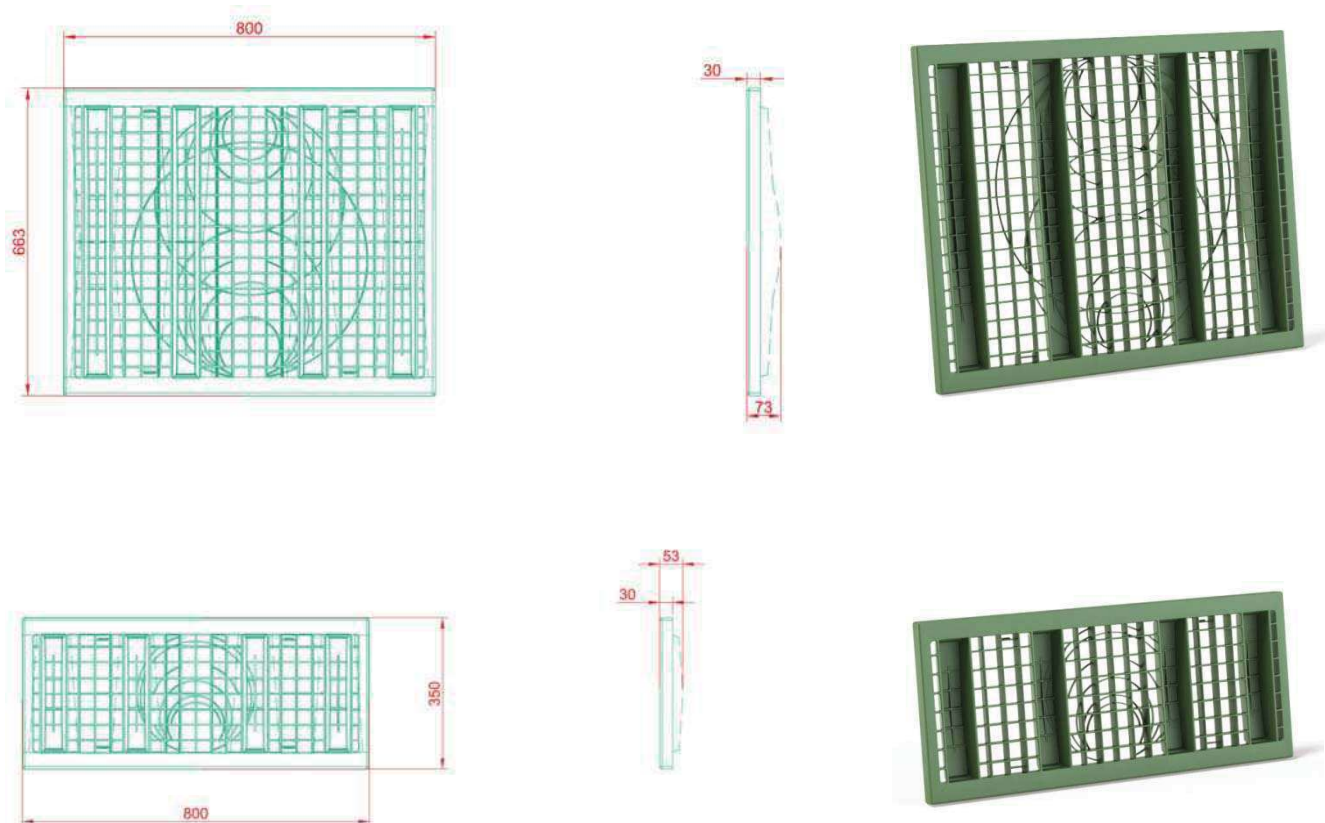
Figure 3b : Face latérale pour module et demi-module Rigofill ST
