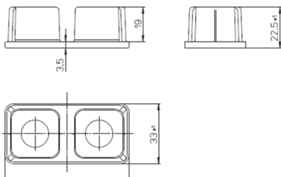
Figure 2 a – Connecteurs monocouches
