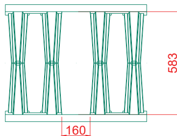
Figure 1e– Caractéristiques dimensionnelles du module Rigofill ST
