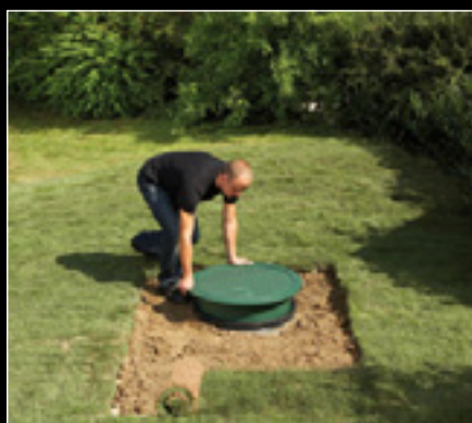
Les photos ci-dessus représentent l'installation d'une cuve Platine® 1500 L.
